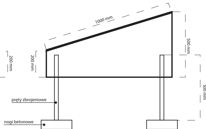
rzut tablicy pamiątkowej z postumentem od boku
